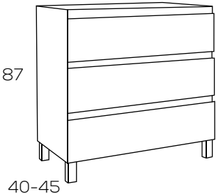
CAJÓN MADERA EXTRACCIÓN PARCIAL PARTIAL-EXTRACTION WOODEN DRAWER / TIROIR EN BOIS EXTRACTION PARTIELLE AMORTIE
