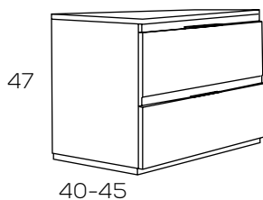
CAJONES METÁLICOS CON EXTRACCIÓN TOTAL FULL-EXTRACTION METALLIC DRAWERS TIROIR EXTENSION COMPLÈTE
