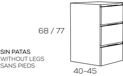
CAJONES METÁLICOS CON EXTRACCIÓN TOTAL FULL-EXTRACTION METALLIC DRAWERS TIROIR EXTENSION COMPLÈTE
